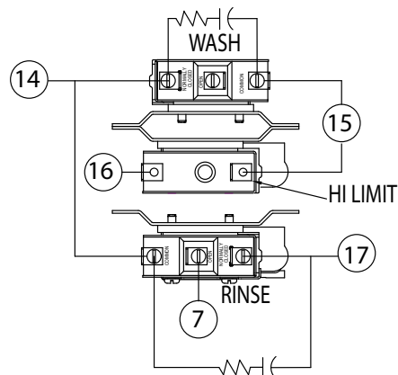
100069 Wiring
